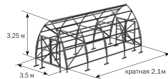
«ФЕРМЕР-3,5» ТЕПЛИЦА
