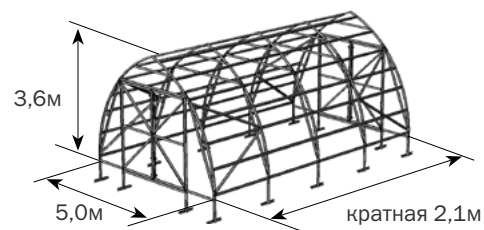
«ФЕРМЕР-5,0» ТЕПЛИЦА
